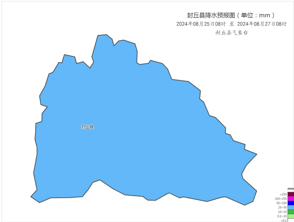
图1 2024年8月25日08时至27日08时封丘县降水预报图（单位：mm）
